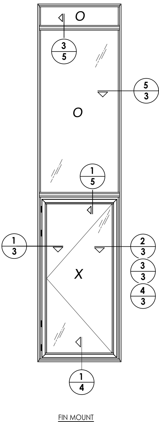
FIN MOUNT
